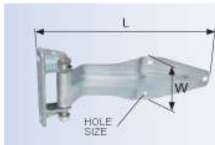
Rear Door Hinge c/w Bracket
