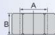
Wheel Nut - Model B DIN 934
